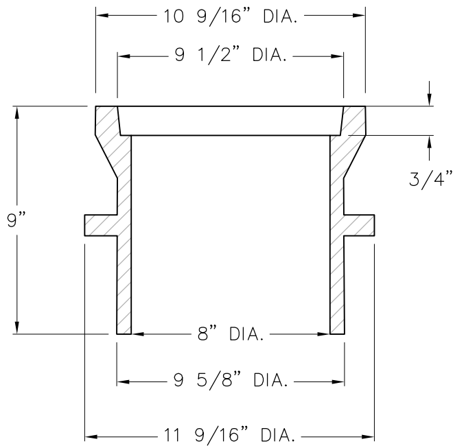
LID SECTION
